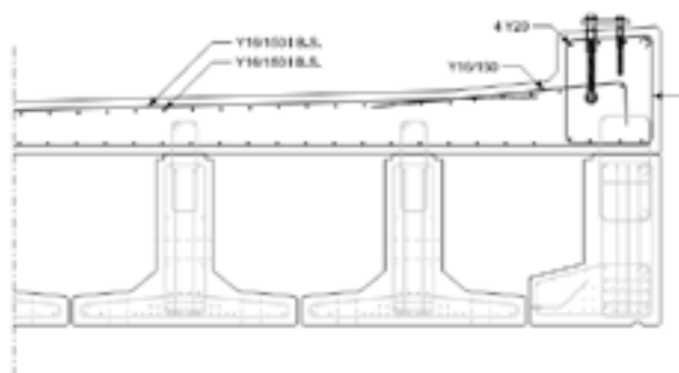
Tværsnit af vejbro. Elementerne forinden produceres i Genner. Ovenpå elementerne ses betonen, der støbes direkte på pladsen, når elementerne er monteret.
